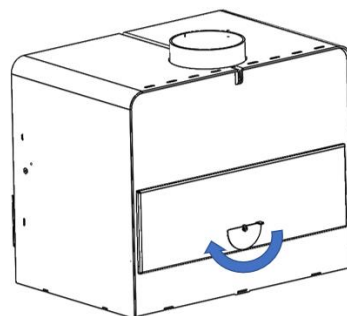
Figure n°8 - Registre d'arrivée d'air de double combustion fermé
