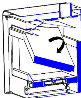
Figure n°11 - Extraction des déflecteurs en vermiculite
