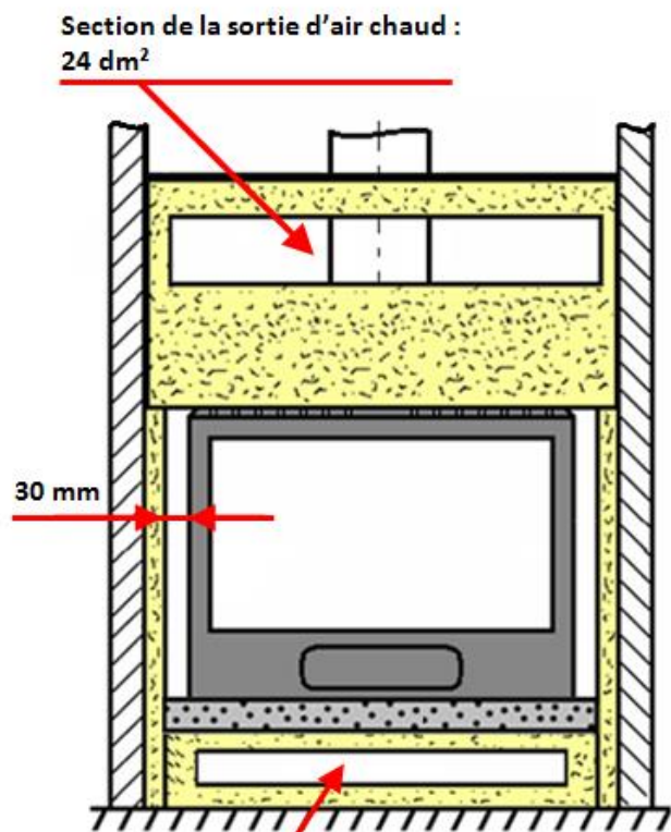
Section de l'entrée d'air frais: 8 dm 2
