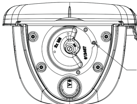
CHC M6x10
