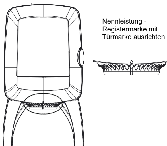
Position „Nennleistung“
