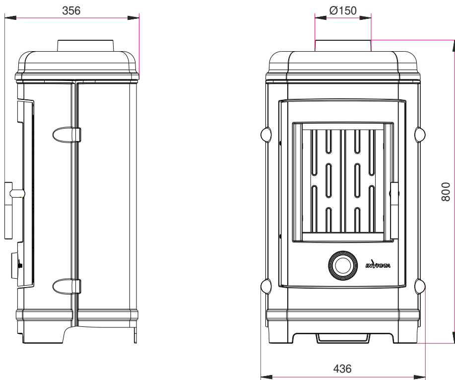
Schéma 2 : Dimensions produits / Product dimensions
